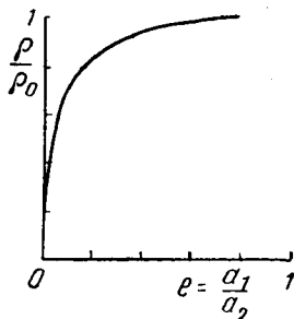
Рис. V. 13. Вспомогательный график для расчета притока к эллиптическому отверстию.
