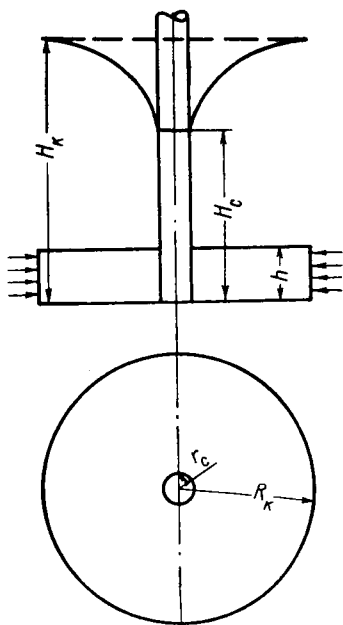
Рис. I. 7. Схема плоско-радиального притока к совершенной скважине.
