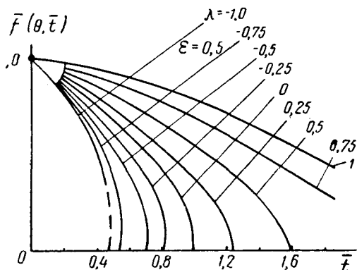
Рис. VII. 8. Графики для расчета времени прорыва воды в скважину, эксцентрично расположенную в круговом пласте, при различных соотношениях вязкостей.
