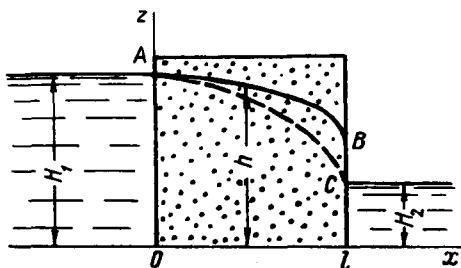
Рис. VI. 1. Схема безнапорного течения через проницаемую перегородку при горизонтальном непроницаемом основании.
