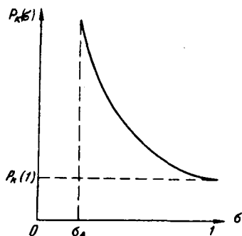
Рис. IX. 2. График зависимости капиллярного давления от насыщенности.
