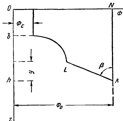
Рис. VII. 15. Распределение потенциала вдоль стенки скважины, ее продолжения и поверхности водяного конуса.
