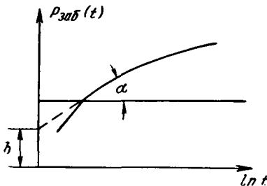
Рис. VIII. 13. График восстановления забойного давления в координатах p_{заб}(t) , \ln t .
