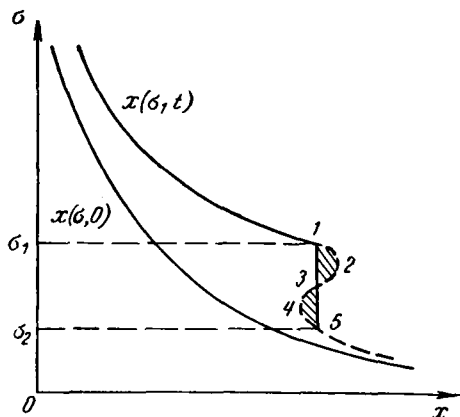
Рис. IX. 6. Устранение многозначности распределения насыщенности введением скачка.
