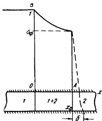
Рис. IX. 7. Распределение насыщенности при вытеснении в пористой среде.
