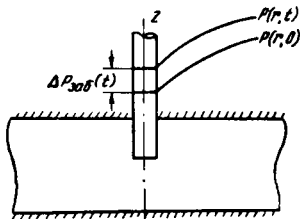
Рис. VIII. 12. График изменения забойного давления после прекращения притока.
