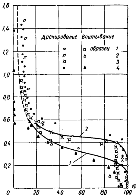
Рис. IX. 3. Графики функции Леверетта.
