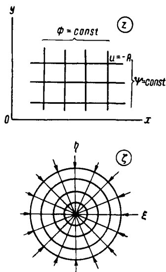
Рис. III. 5. Соответствие между эквипотенциалами и линиями тока при плоско-параллельном течении и притоке к точечному стоку на плоскости.
