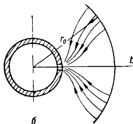
Рис. V. 11. Схема притока к перфорационному отверстию.
