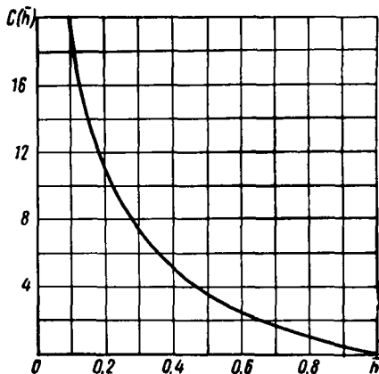
Рис. V. 7. График безразмерного фильтрационного сопротивления для несовершенной скважины без донного притока.
