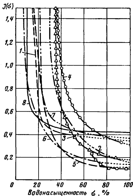
Рис. IX. 4. Кривые капиллярного давления (по Розе и Брусу).
