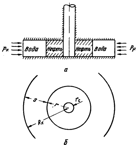
Рис. VII. 12. Схема плоско-радиального движения водо-нефтяного контакта.
