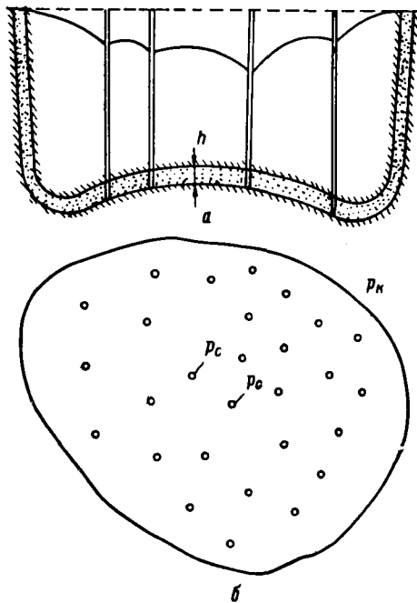
Рис. IV. 1. Схема притока к скважинам при напорном режиме.
